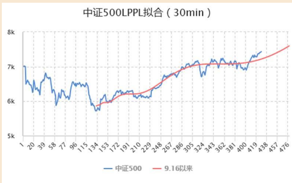
图四 中证500指数30分钟实际走势与拟合效果
