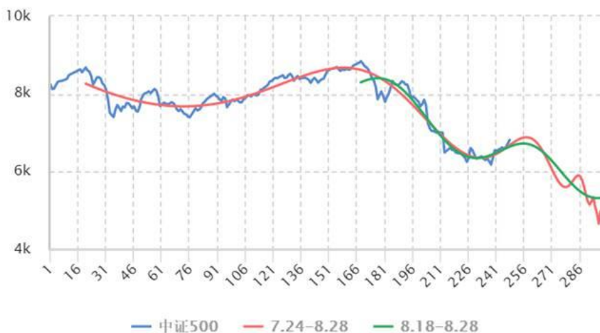
中证500LPPL拟合（30min）
