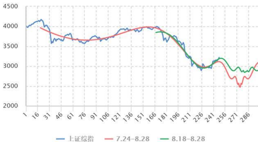
上证综指LPPL拟合（30min）
